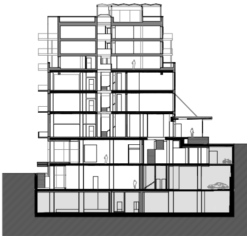
Wohnungsgrundrisse im fünften Stock (oben) und Querschnitt.
